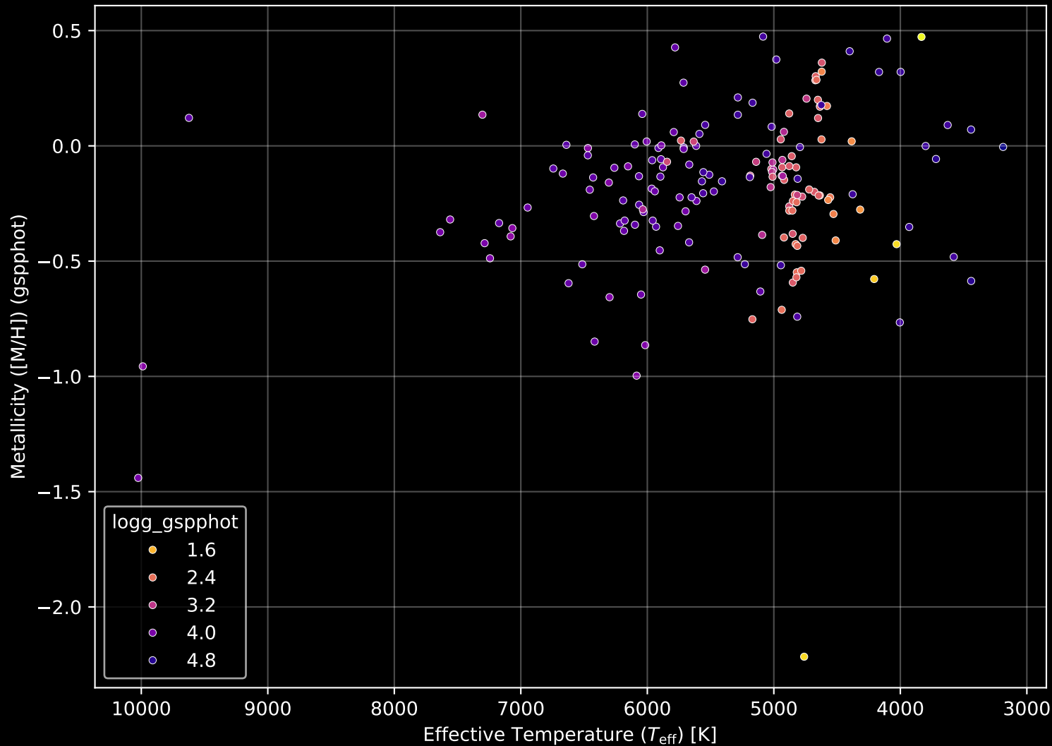
APOGEE DR17 Field: [CVZTILE_086+27_btx] Stellar Population Parameters (n= 173)
